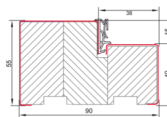
ościeżnica stalowo drewniana (za dopłatą)
